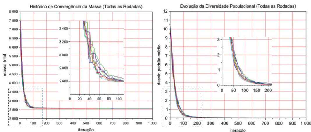
Figura 8 - Gráficos referentes ao histórico de convergência e evolução da diversidade populacional para a treliça com 17 barras.
