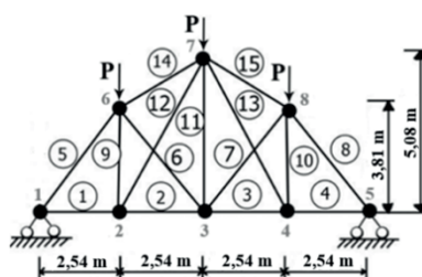
Figura 5 - Modelo estrutural da treliça com 15 barras.
