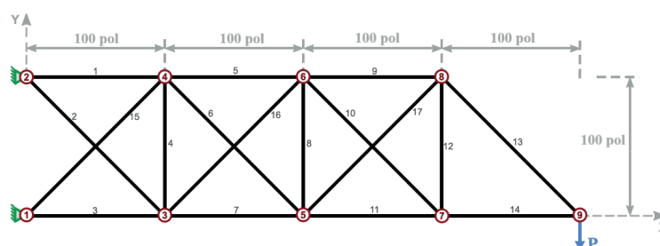
Figura 7 - Modelo estrutural da treliça com 17 barras.
