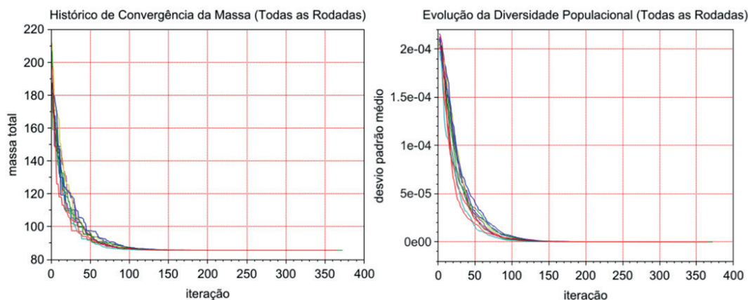
Figura 6 - Gráficos referentes ao histórico de convergência e evolução da diversidade populacional para a treliça com 15 barras.
