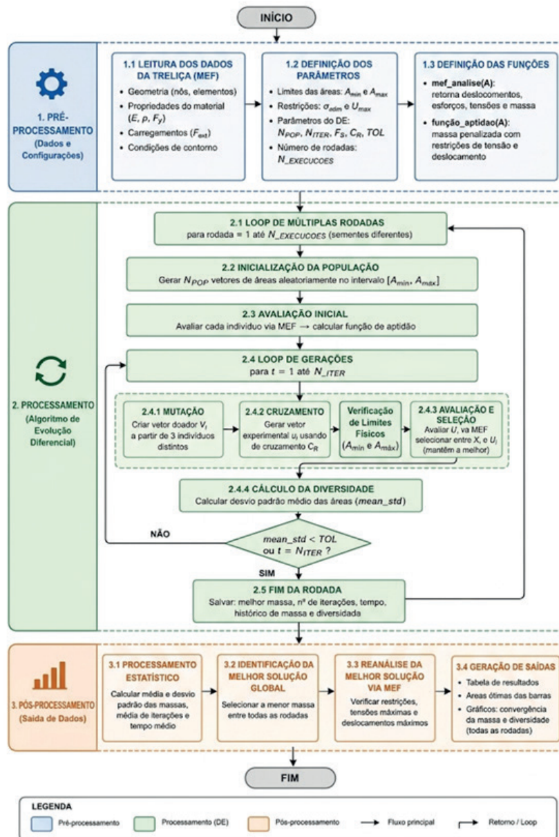
Figura 1 - Pseudocódigo do algoritmo de otimização estrutural via DE acoplada ao MEF.
