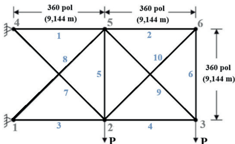
Figura 3 - Modelo estrutural da treliça com 10 barras.
