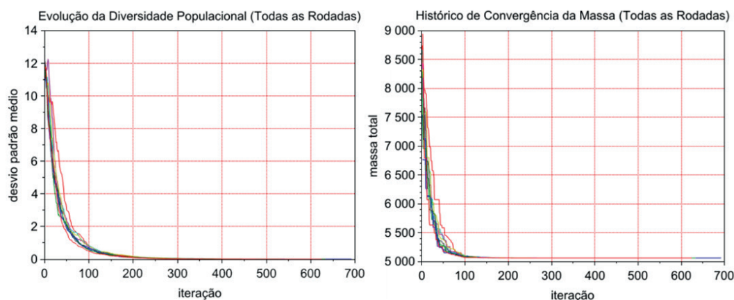
Figura 4 - Gráficos referentes ao histórico de convergência e evolução da diversidade populacional para a treliça com 10 barras.
